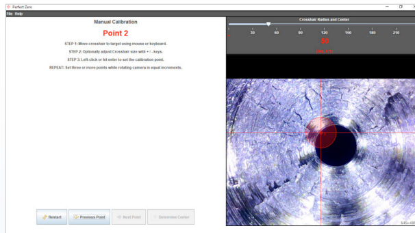
Screenshot der Perfect Zero-Software beim Ausmessen verschiedener Punkte auf dem Werkzeug.
