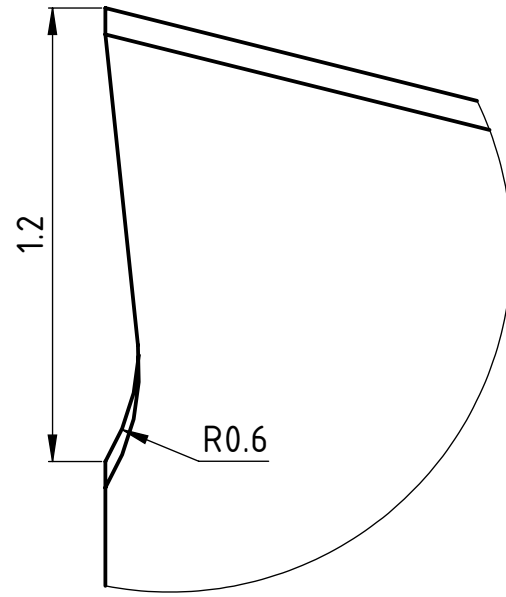
B (50 : 1)
